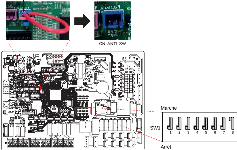
Goupille courte de l'antigel
