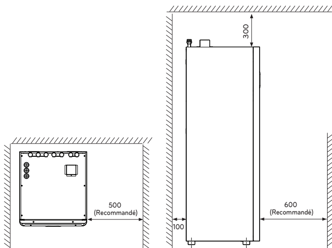
Espace de maintenance minimum (unité : mm)
