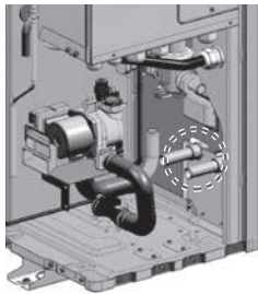
Tuyaux en caoutchouc existants
