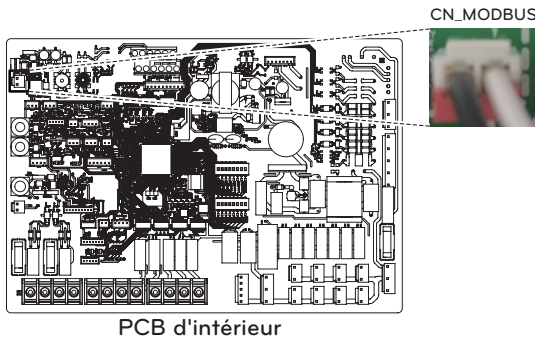
PCB d'intérieur
