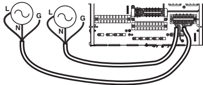
Chauffage d'appoint 1Ø (Pour unité intérieure Split R32 série 4)
