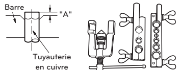
<Type d'embrayage>
