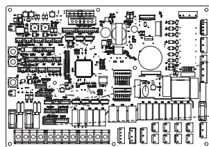
PCB d'intérieur
