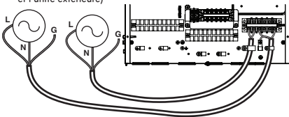
Chauffage d'appoint 1Ø (pour Hydrosplit)
