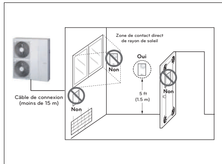
Capteur de température d'air à distance
