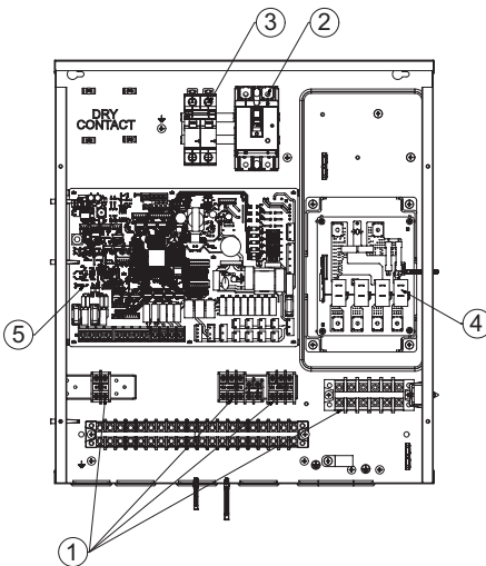
Modèle de chauffage électrique 1Ø (Pour l'unité intérieure R32 Série 5, Pour l'unité intérieure R410A Série 5)
