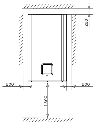
Espacio de servicio (unidad : mm)
