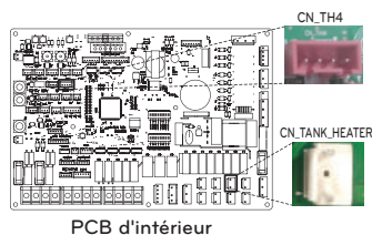
(Pour l'unité intérieure Split Série 5, Pour Hydrosplit)
