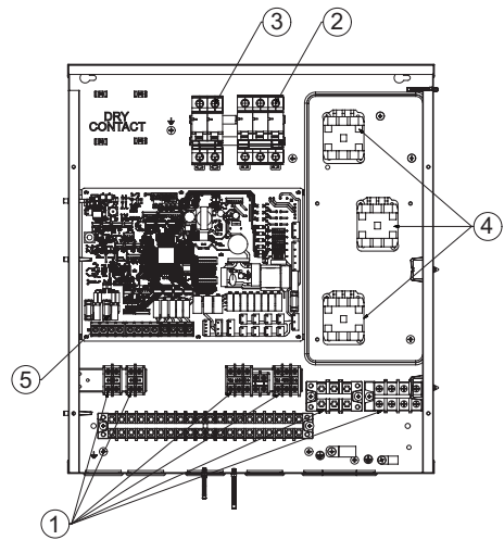
Modèle de chauffage électrique 3Ø (Pour l'unité intérieure R410A série 5)
