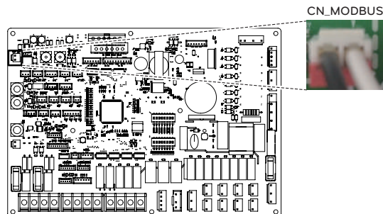
PCB d'intérieur
