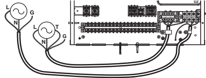
Chauffage d'appoint 3Ø (Pour unité intérieure Split R410A série 5)
