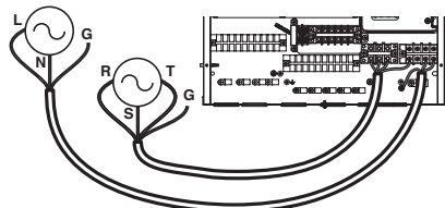
Chauffage d'appoint 3Ø (Pour unité intérieure Split R410A série 3)
