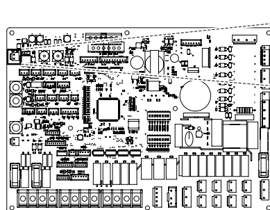
PCB d'intérieur
