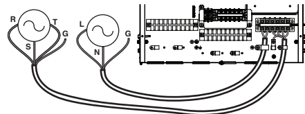
Chauffage d'appoint 3Ø (pour Hydrosplit)
