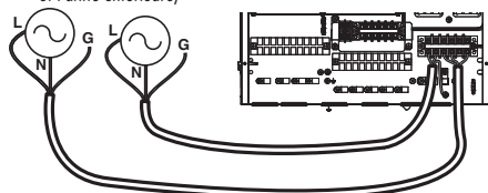
Chauffage d'appoint 1Ø (Pour unité intérieure Split R410A série 3)
