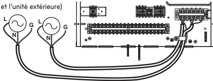
Chauffage d'appoint 1Ø (Pour unité intérieure Split R410A série 5, pour unité intérieure Split R32 série 5)
