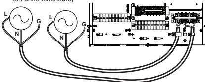
Chauffage d'appoint 1Ø (pour Hydrosplit)
