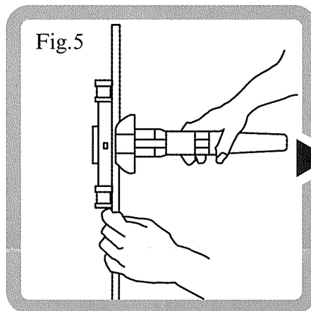
Insérer le tube suivant la même direction que la barre et dépla- cer le mandrin jusqu'au bon angle puis baisser la poignée afin d'éjecter le mandrin.
