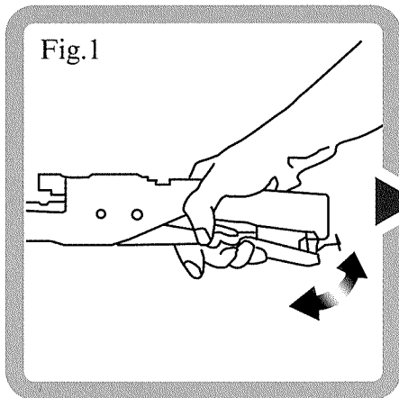
Ejecter la poignée
